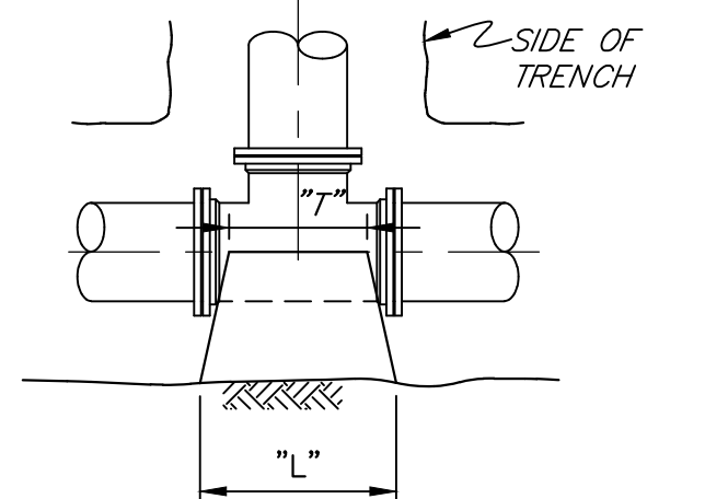
TEE
