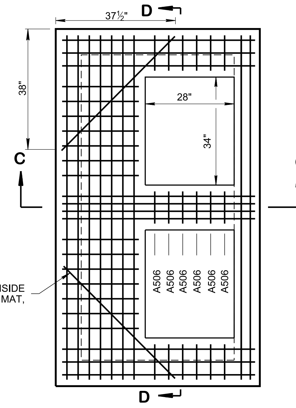
LID REINFORCING
