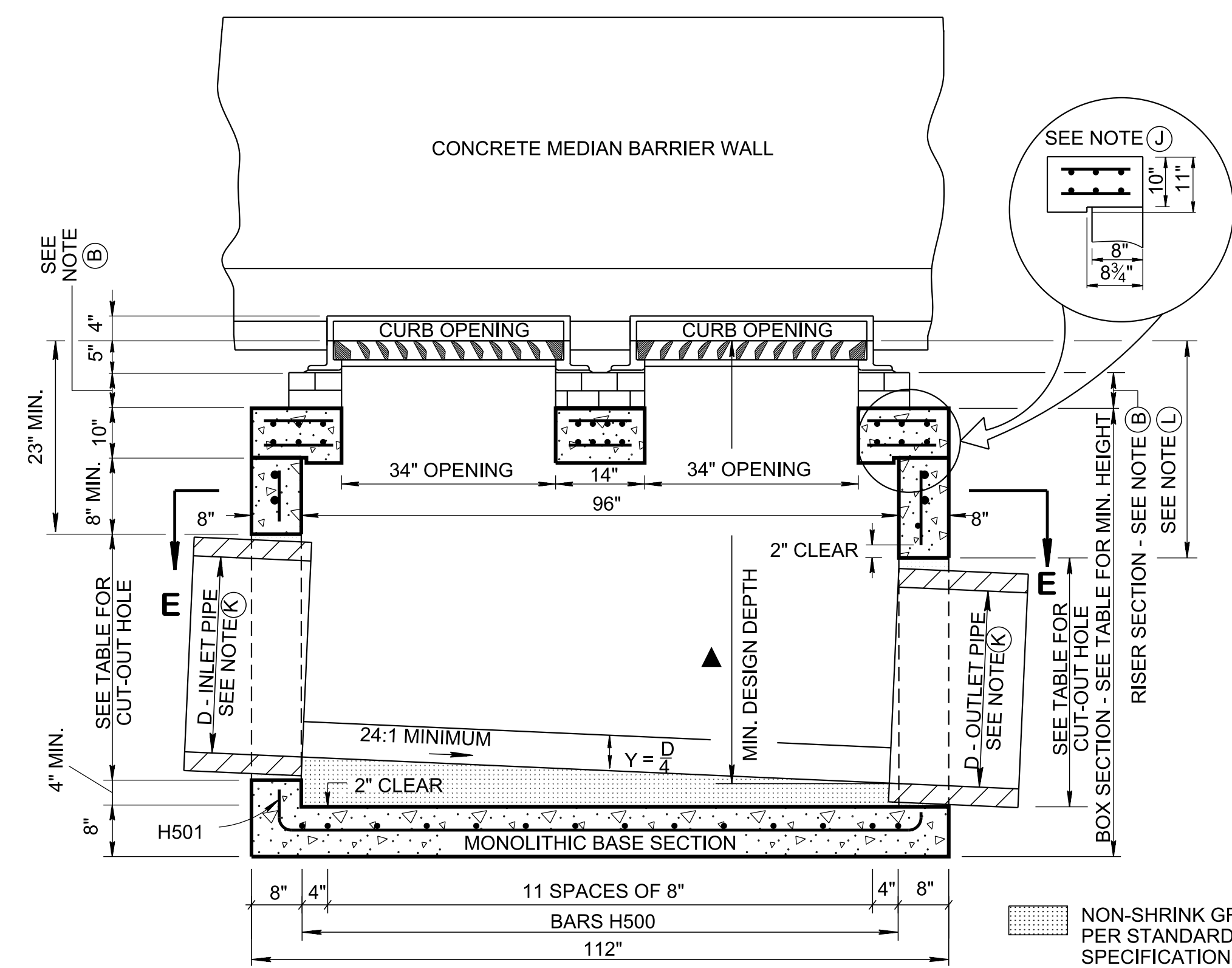
SECTION A-A
