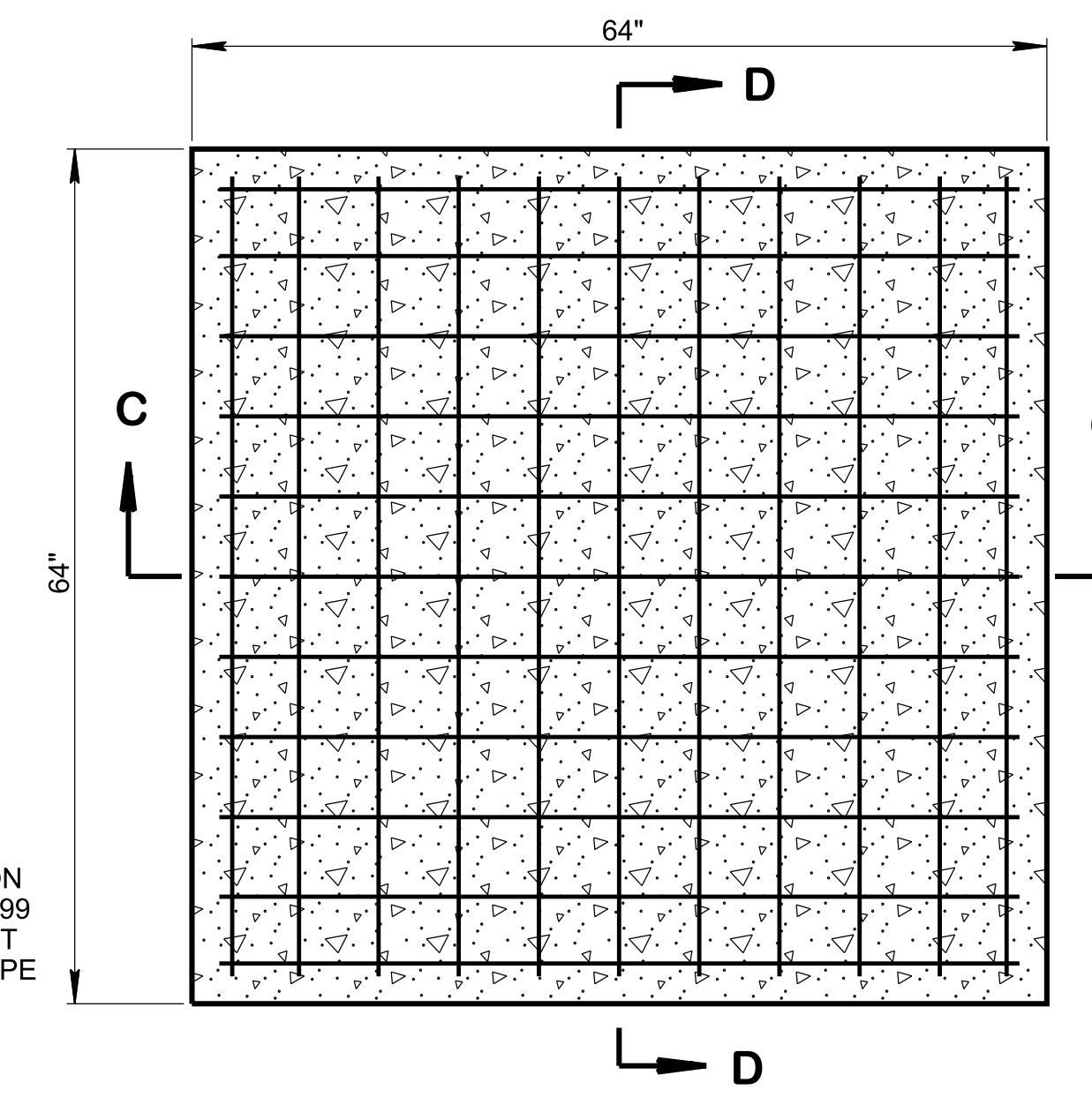
LID REINFORCING
