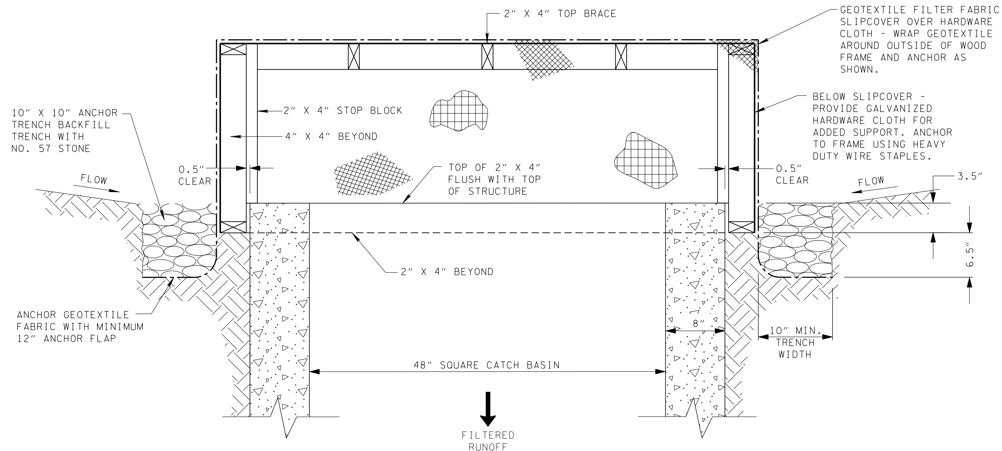
SECTION B-B N.T.S.
