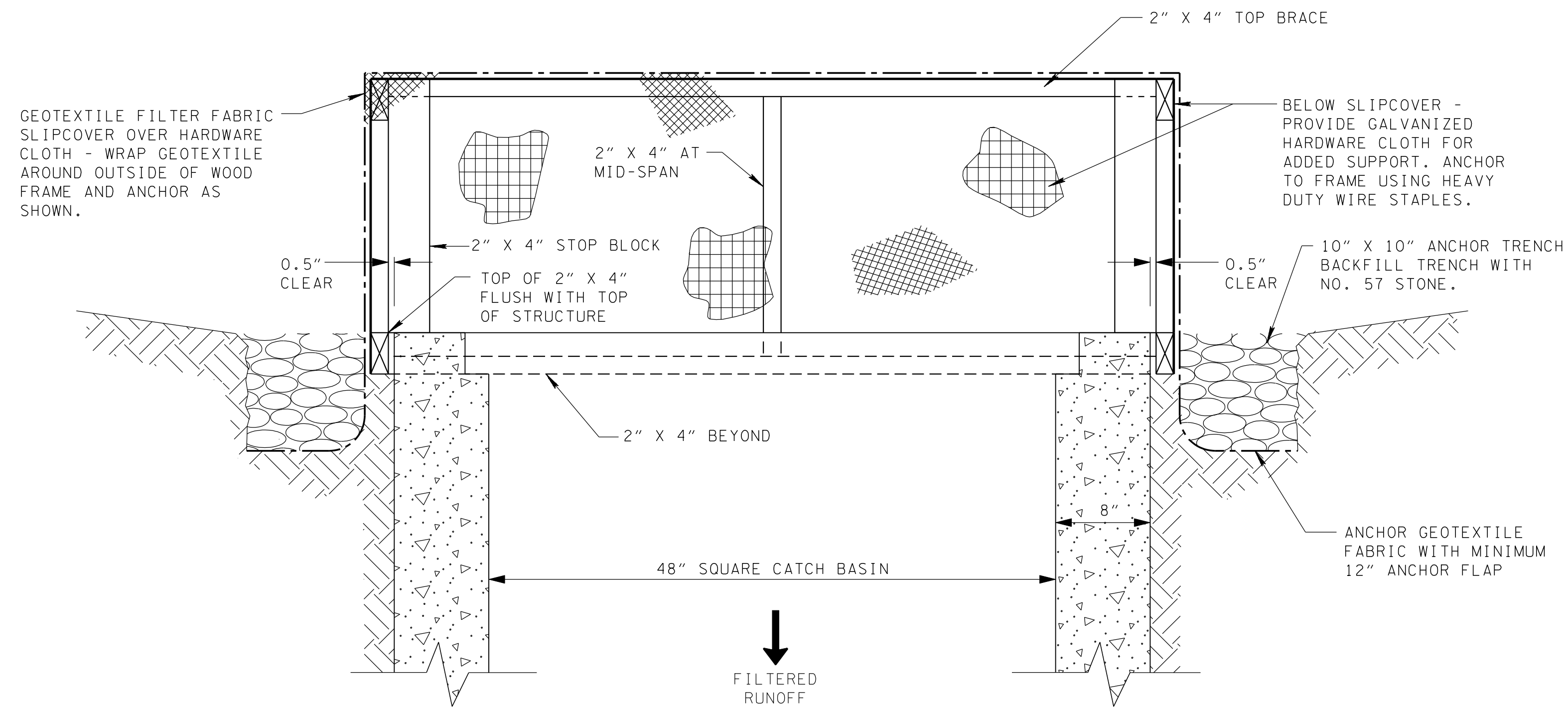
SECTION A-A N.T.S.
